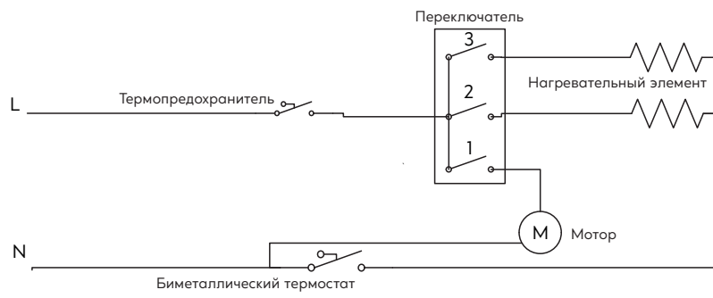
Модели ТР-20R, ТР-30R
