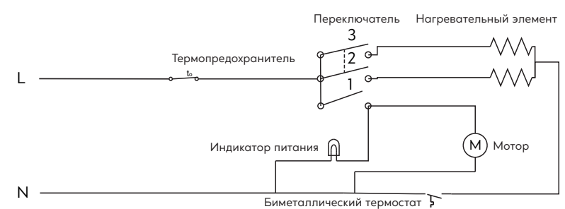
Модели ТРК-20R, ТРК-30R, ТРК-20RB, ТРК-30RB
