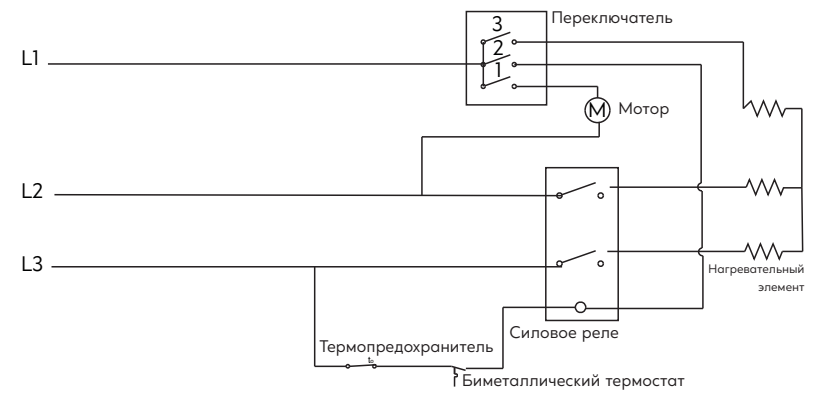
Модели ТР-60R, ТР-90R
