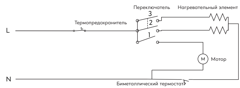
Модели ТРК-20, ТРК-30, ТРК-20В, ТРК-30В
